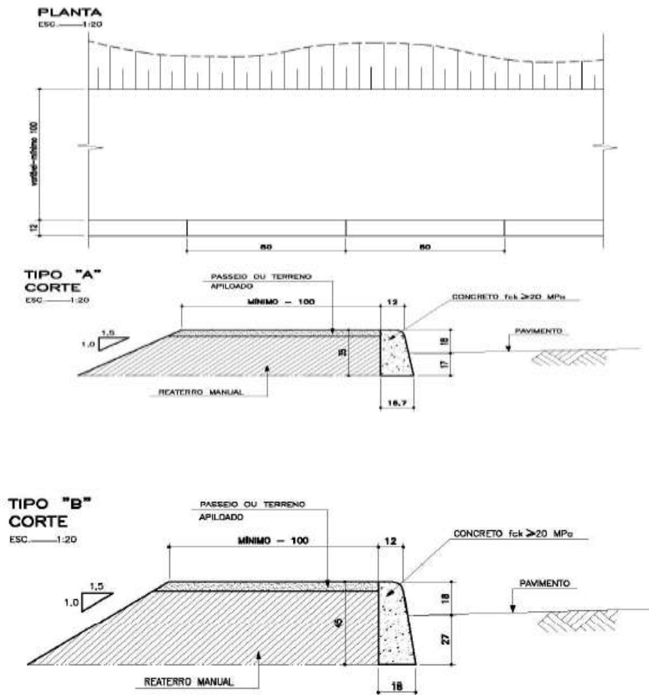
Figura 1 – Detalhe de meio-fio e passeio
