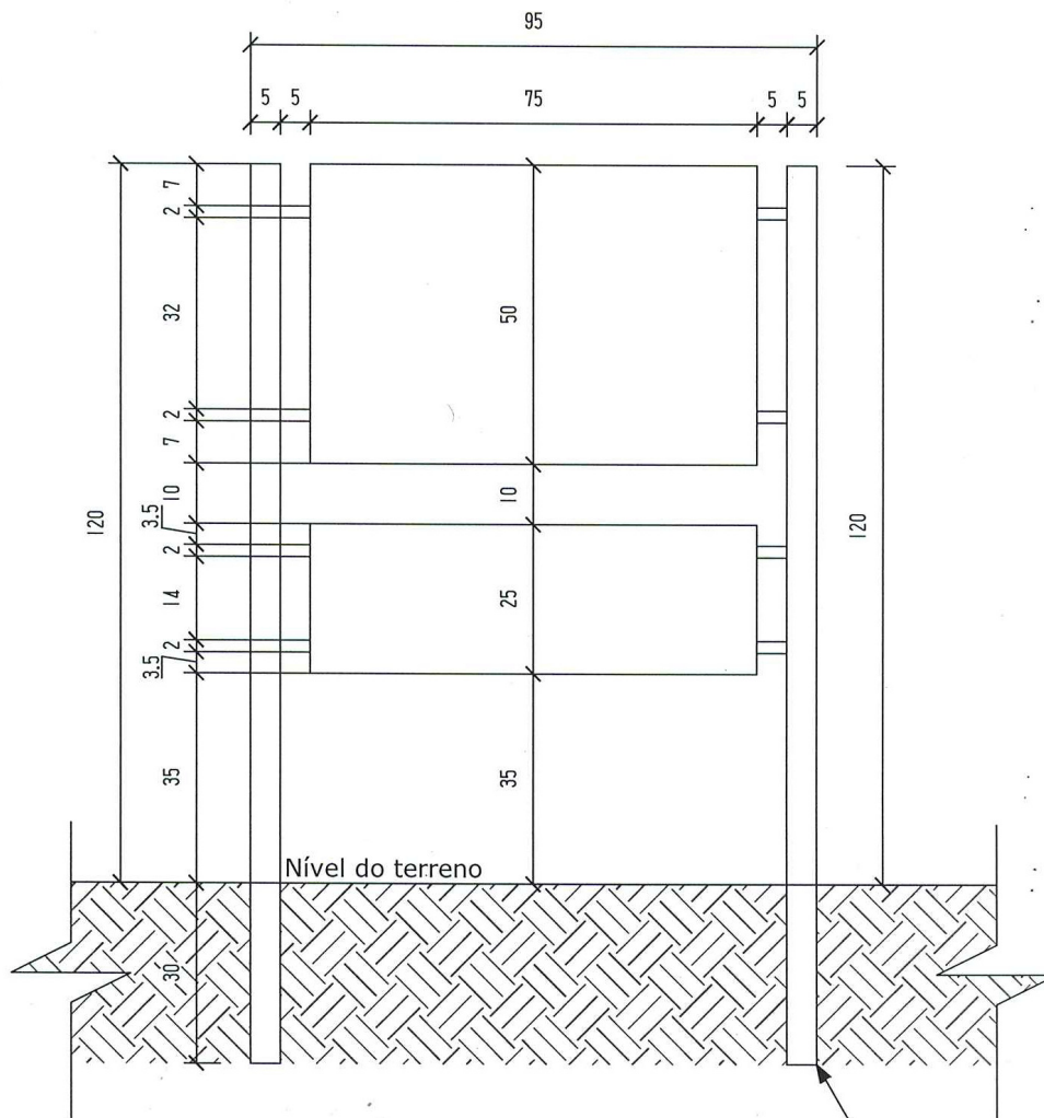
ELEVAÇÃO FRONTAL
